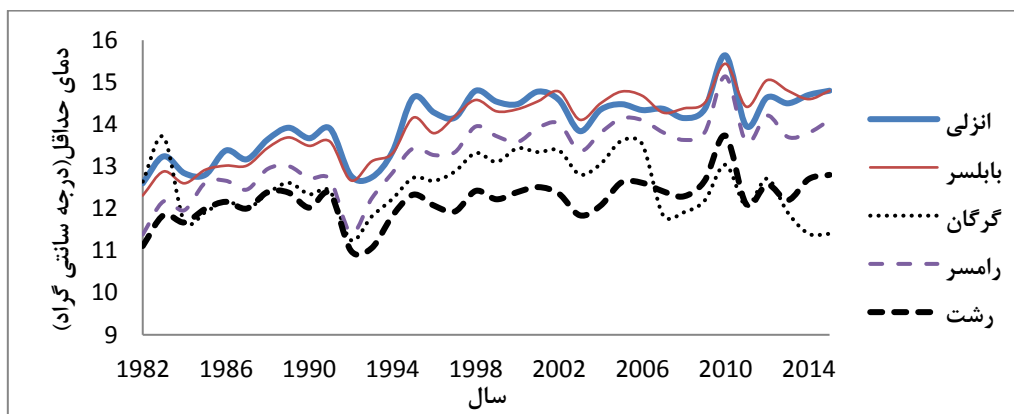
شکل ۱: دمای حداقل دوره مشاهداتی ۱۹۸۲-۲۰۱۵.
