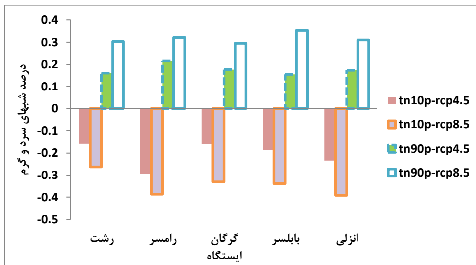
شکل ۶: مقادیر روند شب‌های سرد و گرم در دوره آینده.
