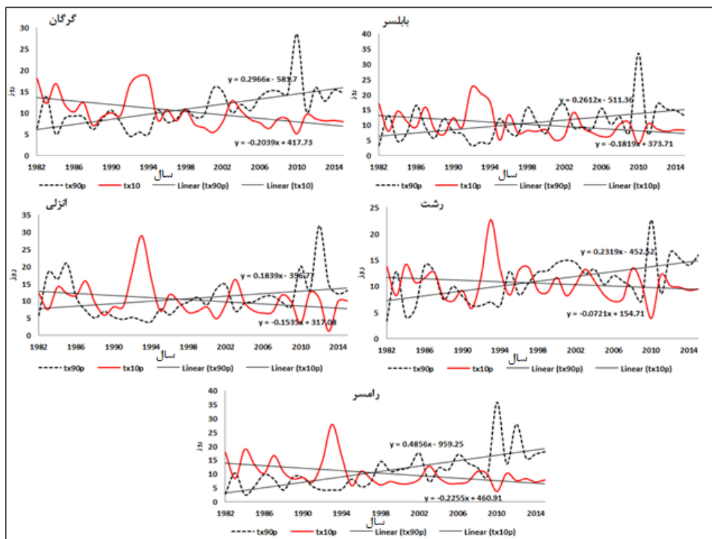
شکل ۷: روند شاخص روزهای سرد و روزهای گرم در دوره مشاهداتی ۲۰۱۵-۱۹۸۲.
