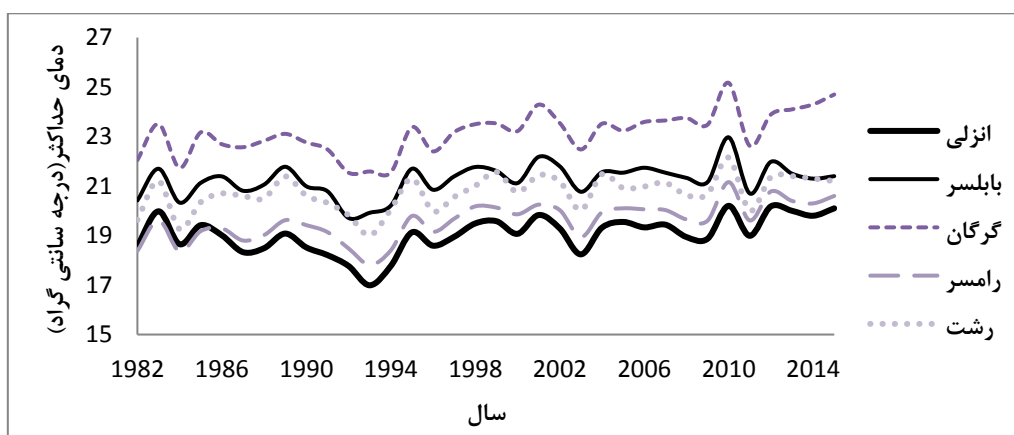
شکل ۲: دمای حداکثر دوره مشاهداتی ۱۹۸۲-۲۰۱۵.
