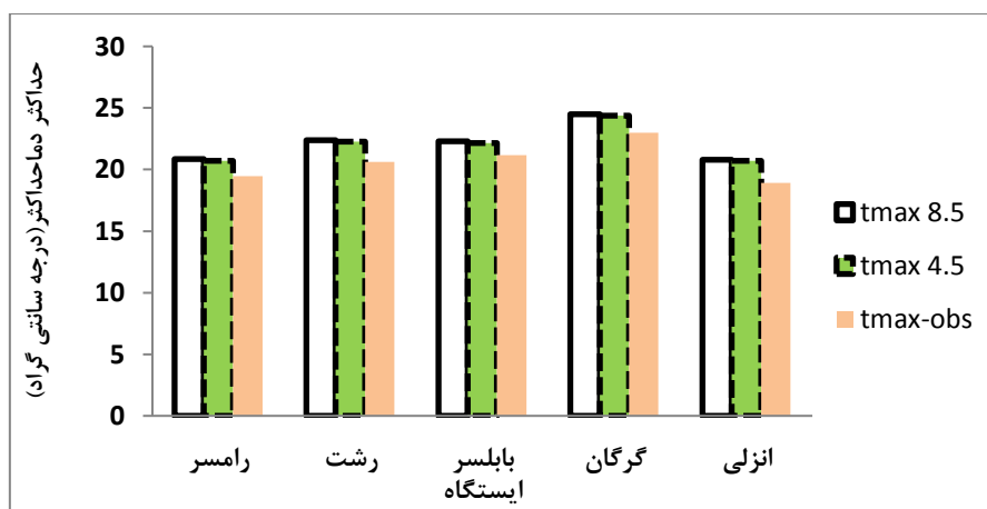
شکل ۴: تغییرات دمای حداکثر ایستگاه‌های مورد مطالعه برای دوره‌های مشاهداتی و تولید شده.
