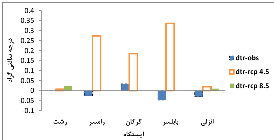
شکل ۹: روند شاخص دامنه تغییرات شبانه روزی دما در دوره حاضر و آینده.
