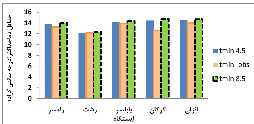
شکل ۳: تغییرات دمای حداقل ایستگاه‌های مورد مطالعه برای دوره‌های مشاهداتی و تولید شده.
