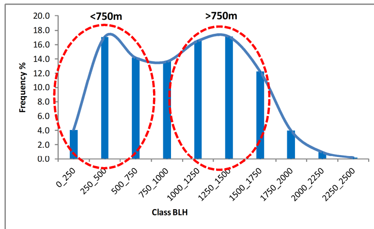
شکل ۲: توزیع فراوانی وقوع ارتفاع لایه مرزی در موقعیت‌های شهری استان اصفهان (۲۰۱۹-۲۰۲۲).
