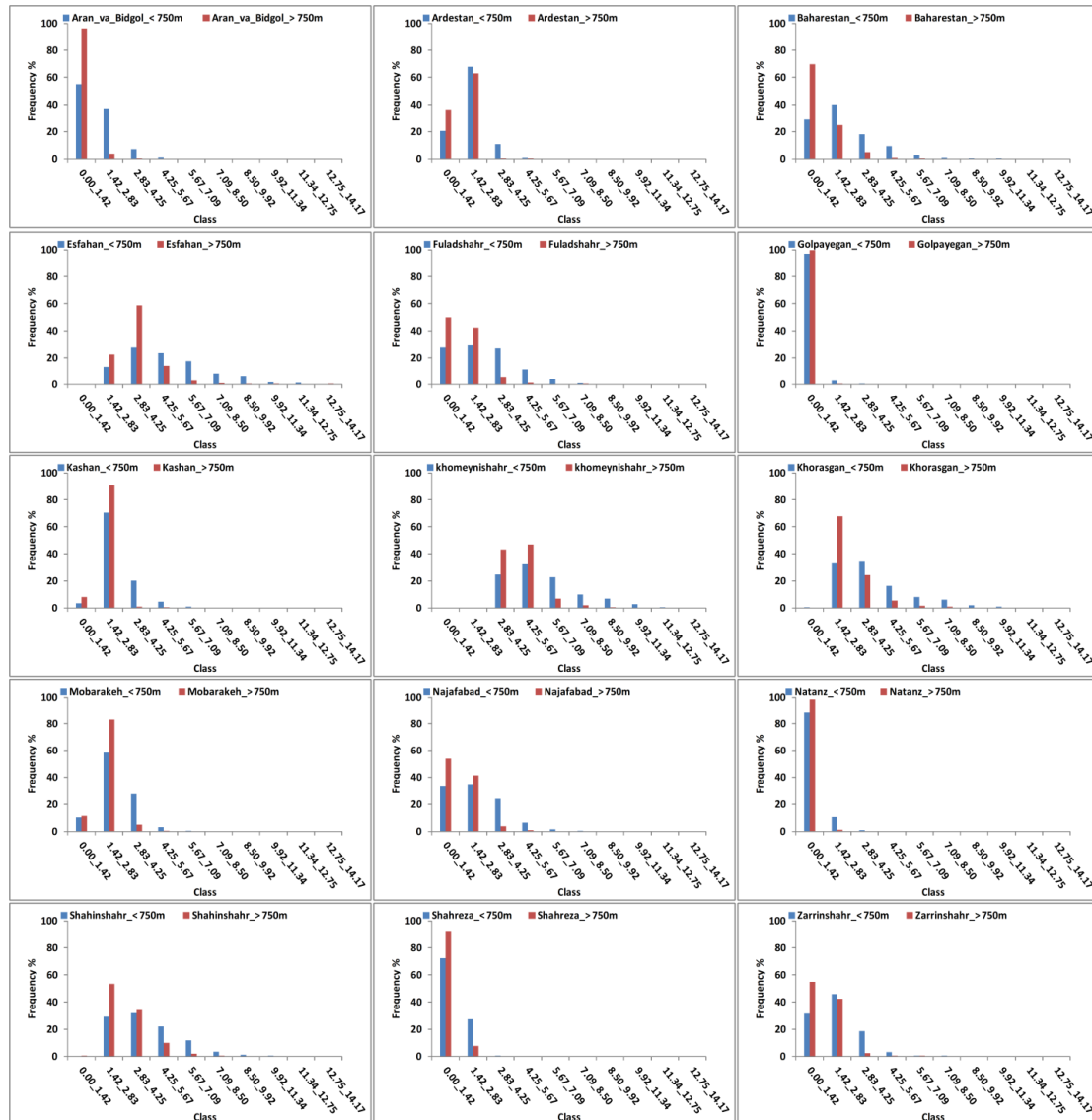
شکل ۴: مقایسه فراوانی وقوع شدت دی اکسید نیتروژن NO2 همزمان با ارتفاع لایه مرزی پایین تر و بالاتر از ۷۵۰ متری.
