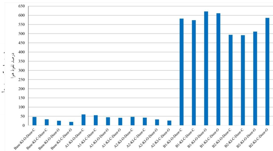
شکل ۱۸: نمودار درصد میزان نفوذ هوای الگوها در دوره گرم سال (مأخذ: نگارندگان)
