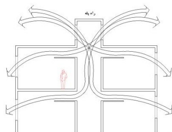
شکل ۶: تاثیر اثر دودکشی فضای ارتباطی عمودی (Murakami et al., 2004)
