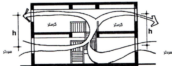
شکل ۳: تأثیر دودکشی راه پله در یک ساختمان دوطبقه (Givoni, 1998).
