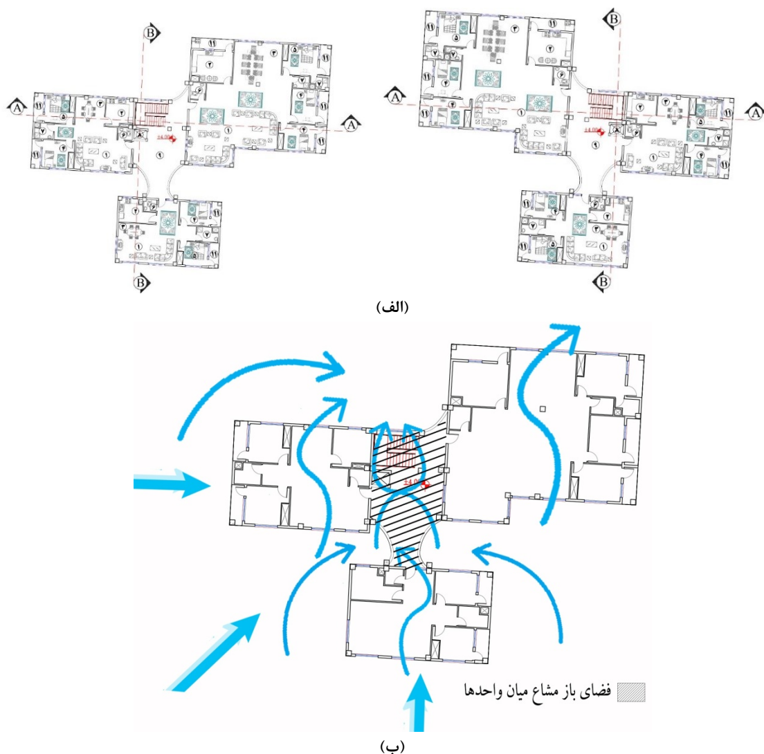
شکل ۱۵: الف) پلان الگوهای B1 و B2 ب) مسیر نفوذ هوا در پلان الگوی B1 (مأخذ: نگارندگان)
