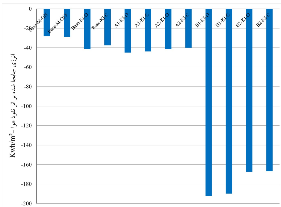
شکل ۱۷: نمودارمیزان مصرف انرژی ناشی از نفوذ هوا در تمام الگوها در حالت درهای باز در دوره گرم سال (مأخذ: نگارندگان)
