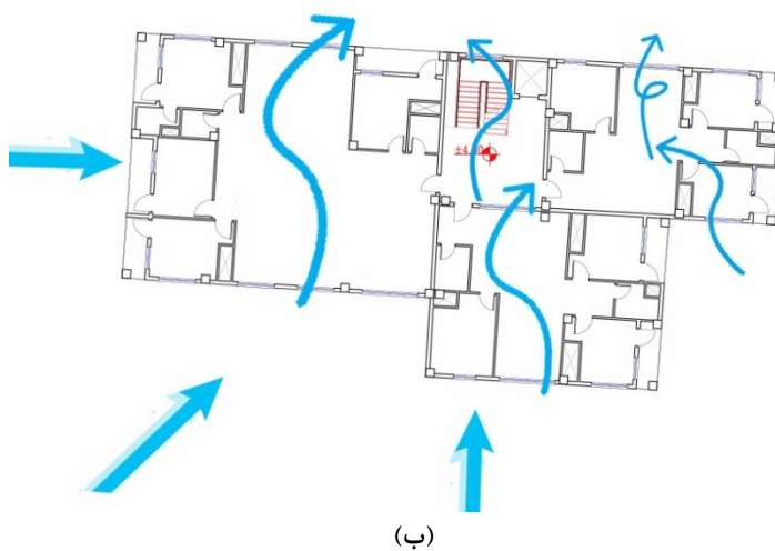
شکل ۱۳: (الف) پلان الگوی Base (ب) مسیر نفوذ هوا در پلان الگوی Base (مأخذ: نگارندگان)
