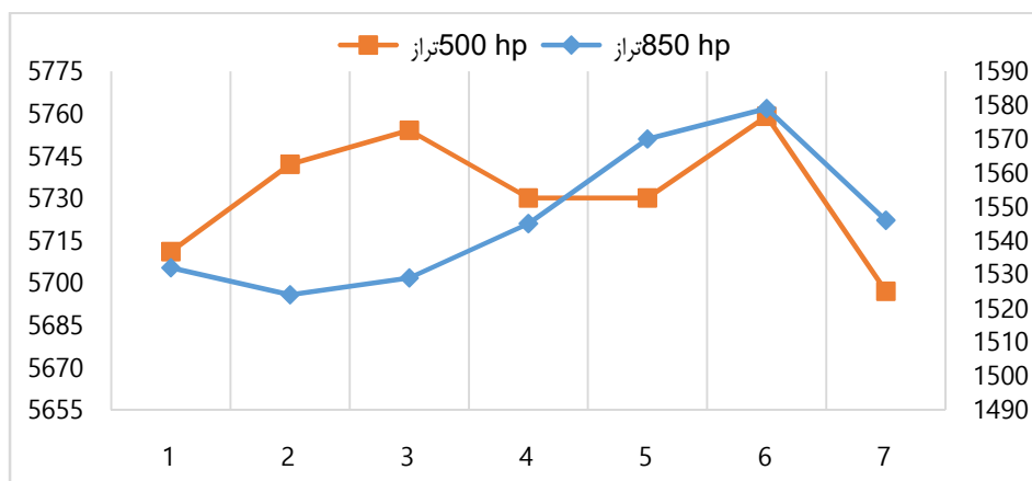
شکل ۱۲: نمودار هافمولر ایستگاه کرمانشاه ۲ تا ۸ ژانویه ۱۹۹۵ (محور راست ارتفاع تراز ۵۰۰ هپ و محور چپ ارتفاع تراز ۸۵۰ هپ به متر و محور افقی روزهای دوره بارشی است).
