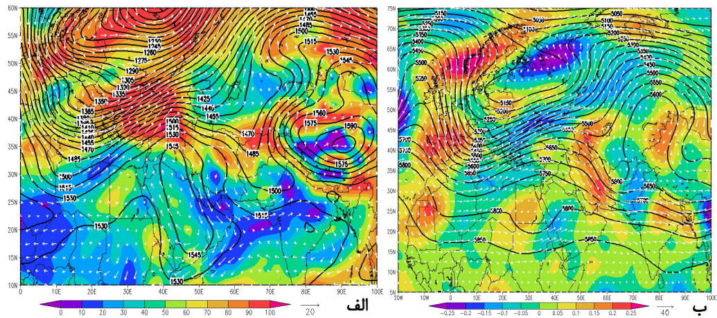
شکل ۱۳: روز دوم تا هشتم ۱۳۹۵ ژانویه: نقشه ارتفاع ژئوپتانسیل (پربند مشکی)، بردار باد (پیکان سفید) و نم‌نسبی (پهنه‌های رنگی) در تراز ۸۵۰ هپ (الف) و ارتفاع ژئوپتانسیل (پربند مشکی)، بردار باد (پیکان سفید) و امگا (پهنه‌های رنگی) در تراز ۵۰۰ هپ (ب).
