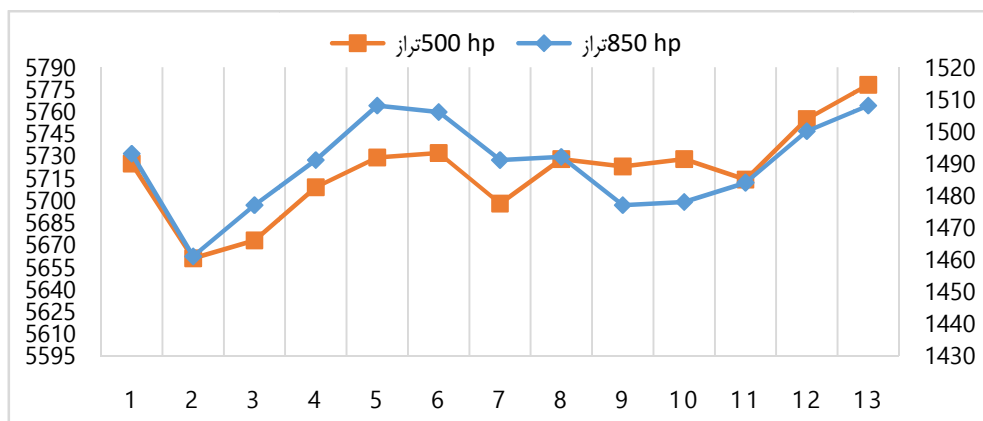
شکل ۱۵: نمودار هاف مولر ایستگاه کرمانشاه ۱۱ تا ۲۳ آوریل ۲۰۰۱ (محور راست ارتفاع تراز ۸۵۰ هپ و محور چپ ارتفاع تراز ۵۰۰ هپ به متر و محور افقی روزهای دوره بارشی است).
