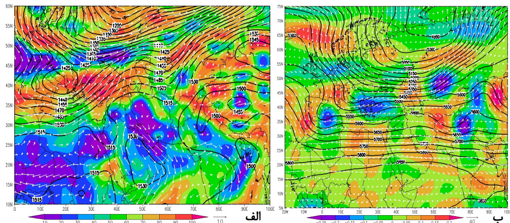
شکل ۱۰: روز ۴ ژانویه ۲۰۰۹: نقشه ارتفاع ژئوپتانسیل (پرند مشکی)، بردار باد (پیکان سفید) و نم‌نسی (پهنه‌های رنگی) در تراز ۸۵۰ هپ (الف) و ارتفاع ژئوپتانسیل (پرند مشکی)، بردار باد (پیکان سفید) و امگا (پهنه‌های رنگی) در تراز ۵۰۰ هپ (ب).
