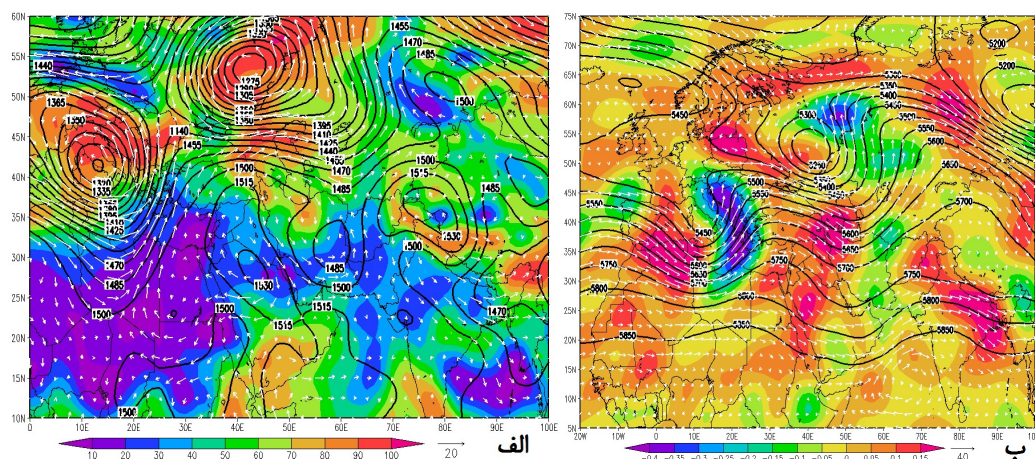
شکل ۱۹: روز ۲۵ تا ۳۱ مارس ۲۰۱۳: نقشه ارتفاع ژئوپتانسیل (پربند مشکی)، بردار باد (پیکان سفید) و نم‌نسبی (پهنه‌های
