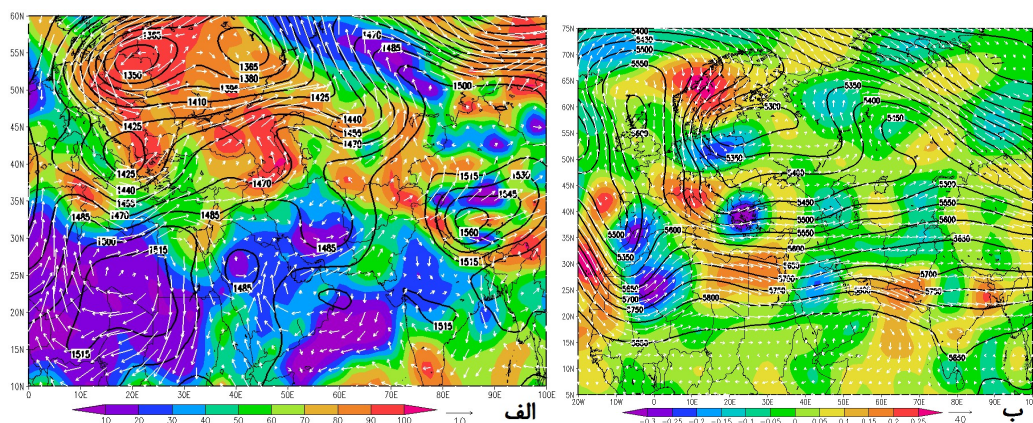
شکل ۱۱: روز ۱۹ فوریه ۲۰۱۳: نقشه ارتفاع ژئوپتانسیل (پرند مشکی)، بردار باد (پیکان سفید) و نم‌نسی (پهنه‌های رنگی) در تراز ۸۵۰ هپ (الف) و ارتفاع ژئوپتانسیل (پرند مشکی)، بردار باد (پیکان سفید) و امگا (پهنه‌های رنگی) در تراز ۵۰۰ هپ (ب).
