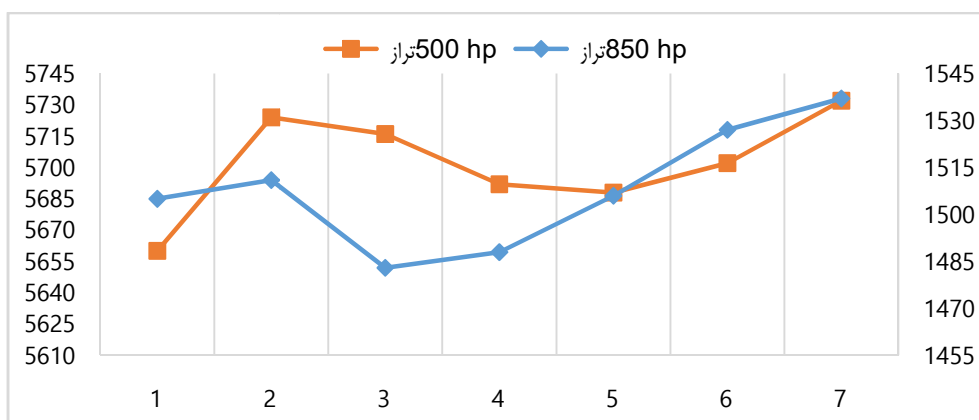
شکل ۱۸: نمودار هافمولر ایستگاه کرمانشاه ۲۵ تا ۳۱ مارس ۲۰۱۳ (محور ۷ سمت راست ارتفاع
