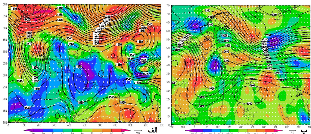
شکل ۸: روز ۱۵ نوامبر ۱۹۹۰: نقشه ارتفاع ژئوپتانسیل (پربند مشکی)، بردار باد (پیکان سفید) و نه‌نسبی (پهنه‌های رنگی) در تراز ۸۵۰ هپ (الف) و ارتفاع ژئوپتانسیل (پربند مشکی)، بردار باد (پیکان سفید) و امگا (پهنه‌های رنگی) در تراز ۵۰۰ هپ (ب).
