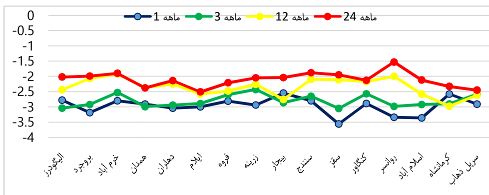
شکل ۷: نمودار بیشینه شدت خشکسالی ها در مقیاس های زمانی مختلف (محور Y شدت SPI)
