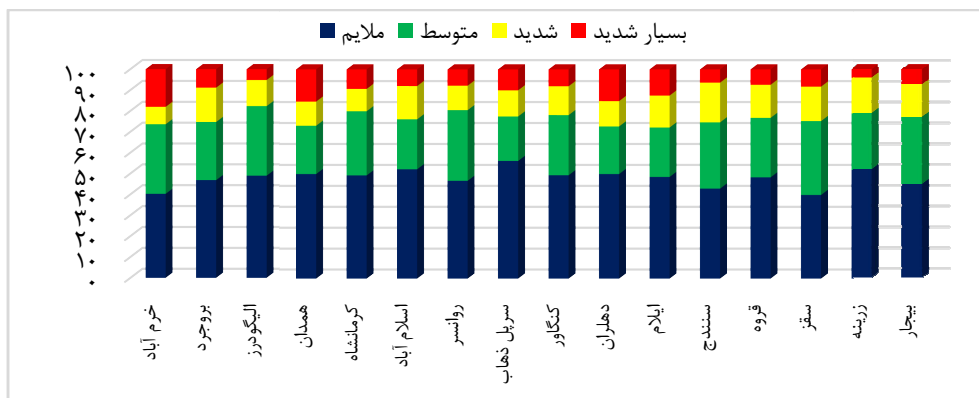
شکل ۴: درصد رخداد خشکسالی به تفکیک شدت‌های مختلف در بازه زمانی ۳ ماهه (محور Y به درصد)
