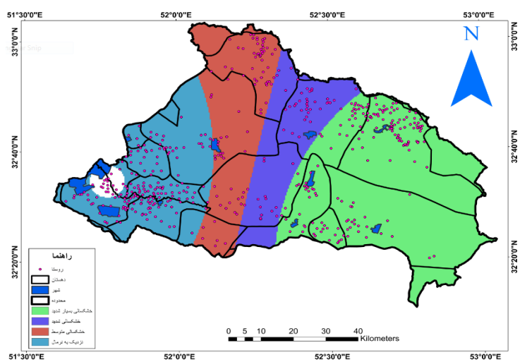
شکل ۱۱: نقشه شاخص خشکسالی SDI در سال ۹۶
