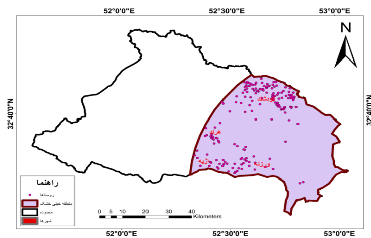
شکل ۱۲: نقشه مناطق در خشکسالی شدید در سال ۹۶
