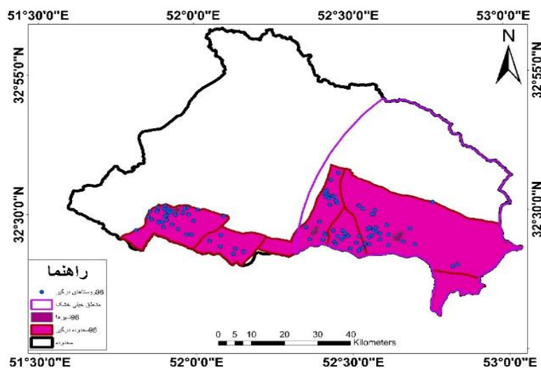
شکل ۱۸: نقشه تطبیقی مناطق بحرانی با تجمعات (SDI) ۱۳۹۶
