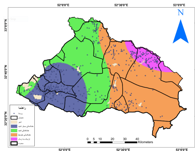
شکل ۳: نقشه شاخص خشک‌سالی SPI در سال ۹۶
