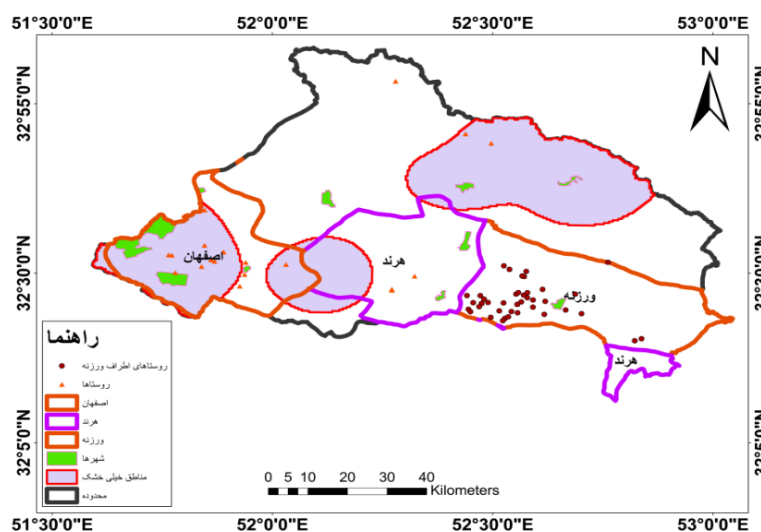
شکل ۱۴: نقشه تطبیقی سال ۱۳۹۱ (SPI)
