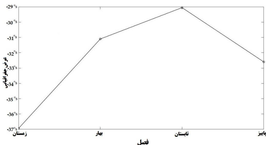
شکل ۷: میانگین تغییرات لبه بیرونی چرخش سلول هادلی نیمکره جنوبی در فصل‌های زمستان، تابستان، بهار و پاییز
