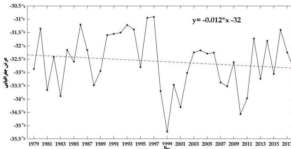
شکل ۳: سری زمانی تغییرات لبه بیرونی چرخش سلول هادلی نیمکره جنوبی در فصل تابستان
