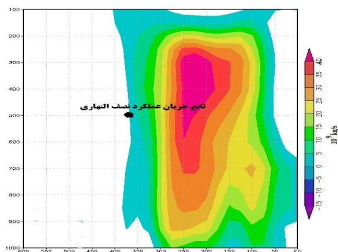
شکل ۱: شماتیک میانگین سالانه چرخش اتمسفری نیمکره جنوبی با موقعیت محاسبات سلول هادلی (۱۹۷۹-۲۰۱۸)، لبه بیرونی تابع جریان عملکرد نصف‌النهاری در تراز 500 \text{ hPa} (دایره مشکی) ( 10^9 \text{ kg/s} )
