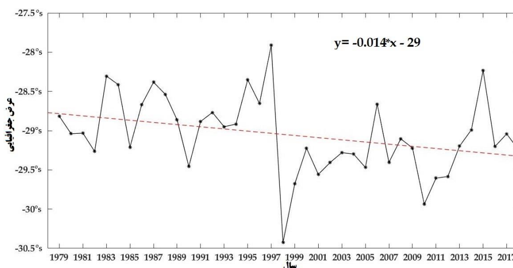
شکل ۴: سری زمانی تغییرات لبه بیرونی چرخش سلول هادلی نیمکره جنوبی در فصل بهار
