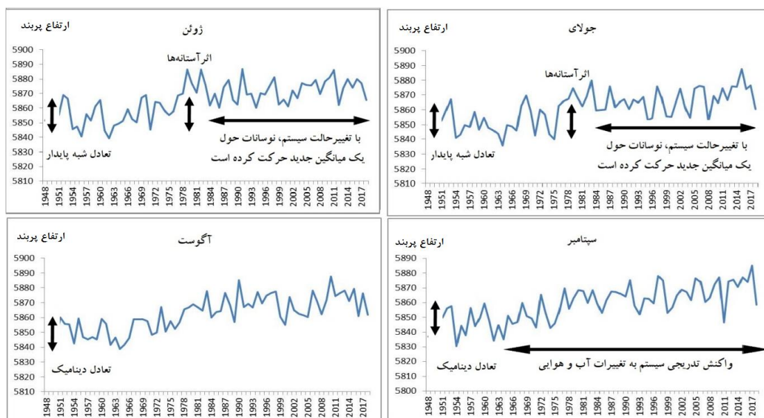
شکل ۵- نمودار افزایش قدرت ارتفاعی بیرونی ترین پربند پراتفاع جنب حاره در دوره مطالعاتی ۱۹۴۸-۲۰۱۸ بر واحد
