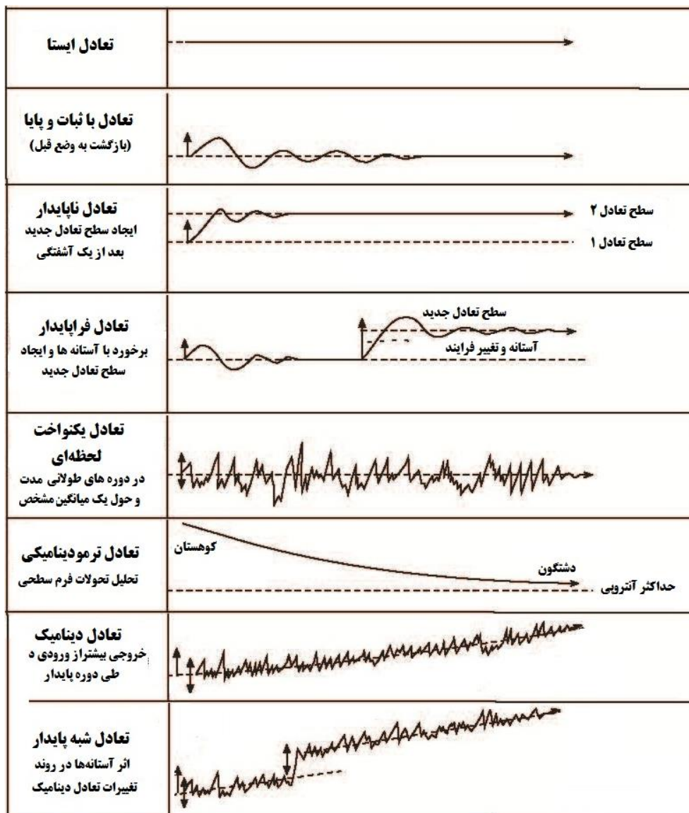
شکل ۱: طبقه بندی تعادل‌های ۸ گانه بر مبنای نظر چورلی و کندی (۱۹۷۱) به نقل از الوردفلدت ۱ ، ۲۰۱۲
