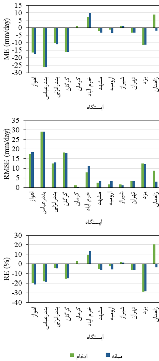
شکل ۶- مقایسه مقادیر شدت بارش ۲۴ ساعته مشاهداتی در هر ایستگاه با روش ادغام و میانہ بر اساس آماره‌های ME، RMSE و RE.
