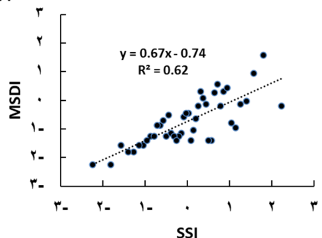
شکل ۹: نمودار پراکنش بین شاخص SSI و SPI (شکل بالا- سمت راست)، شاخص MSDI با SPI (شکل بالا- سمت چپ) و شاخص MSDI با SSI (شکل پایین) در فصل زمستان در ایستگاه گالیکش
