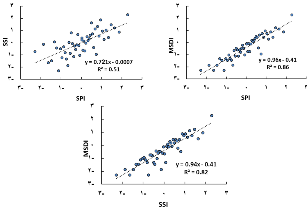
شکل ۲: نمودار پراکنش بین شاخص SSI و SPI (شکل بالا - سمت راست)، شاخص MSDI با SPI (شکل بالا - سمت چپ) و شاخص MSDI با SSI (شکل پایین) در فصل بهار در ایستگاه آرازکوسه
