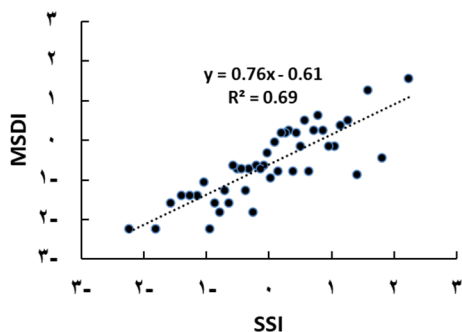
شکل ۸: نمودار پراکنش بین شاخص SSI و SPI (شکل بالا- سمت راست)، شاخص MSDI با SPI (شکل بالا- سمت چپ) و شاخص MSDI با SSI (شکل پایین) در فصل پاییز در ایستگاه گالیکش
